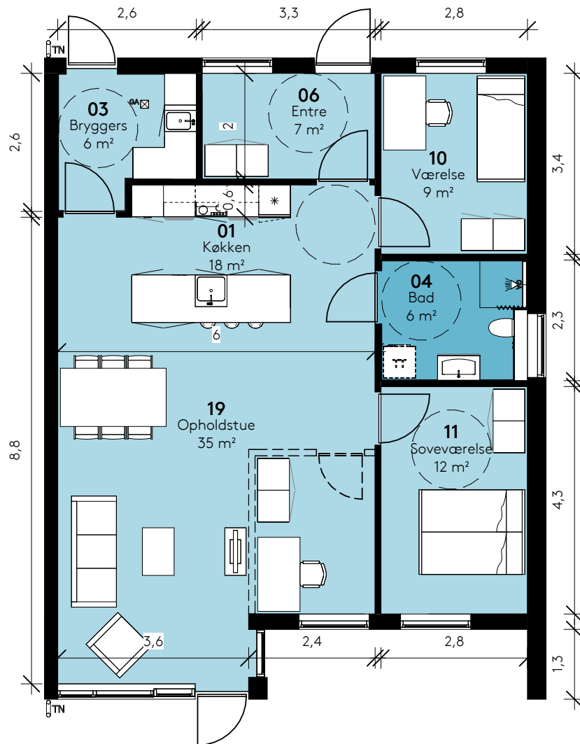
Plan 1 : 100
