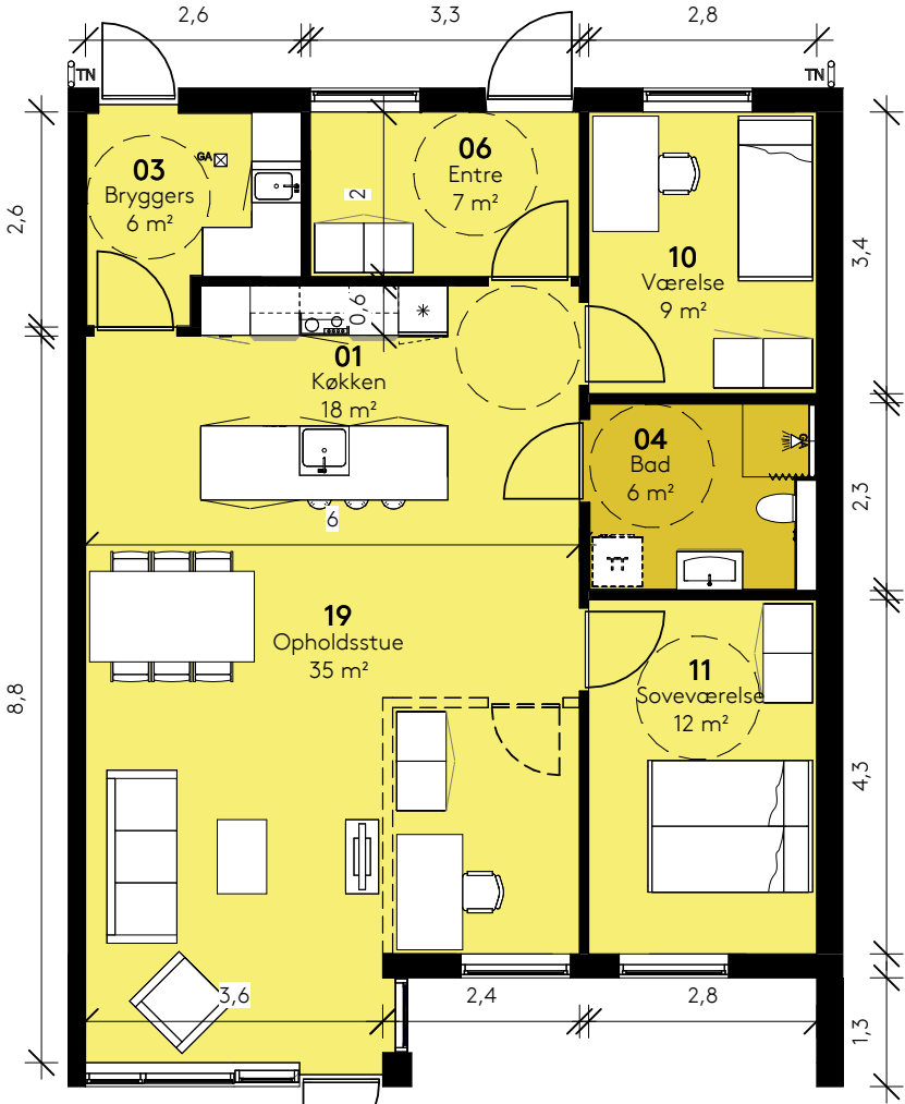
Plan 1 : 100
