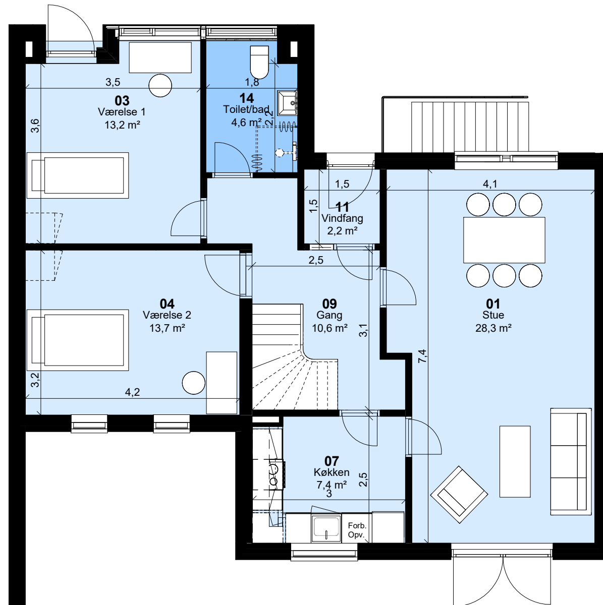
Stueplan
