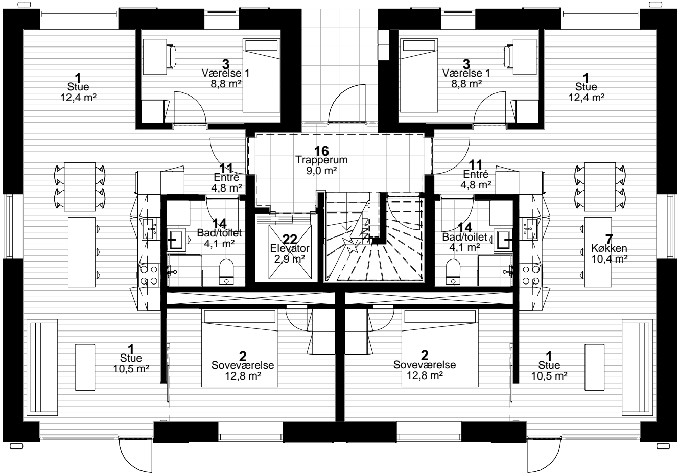
Bygningsplan, stue, bygning 1
